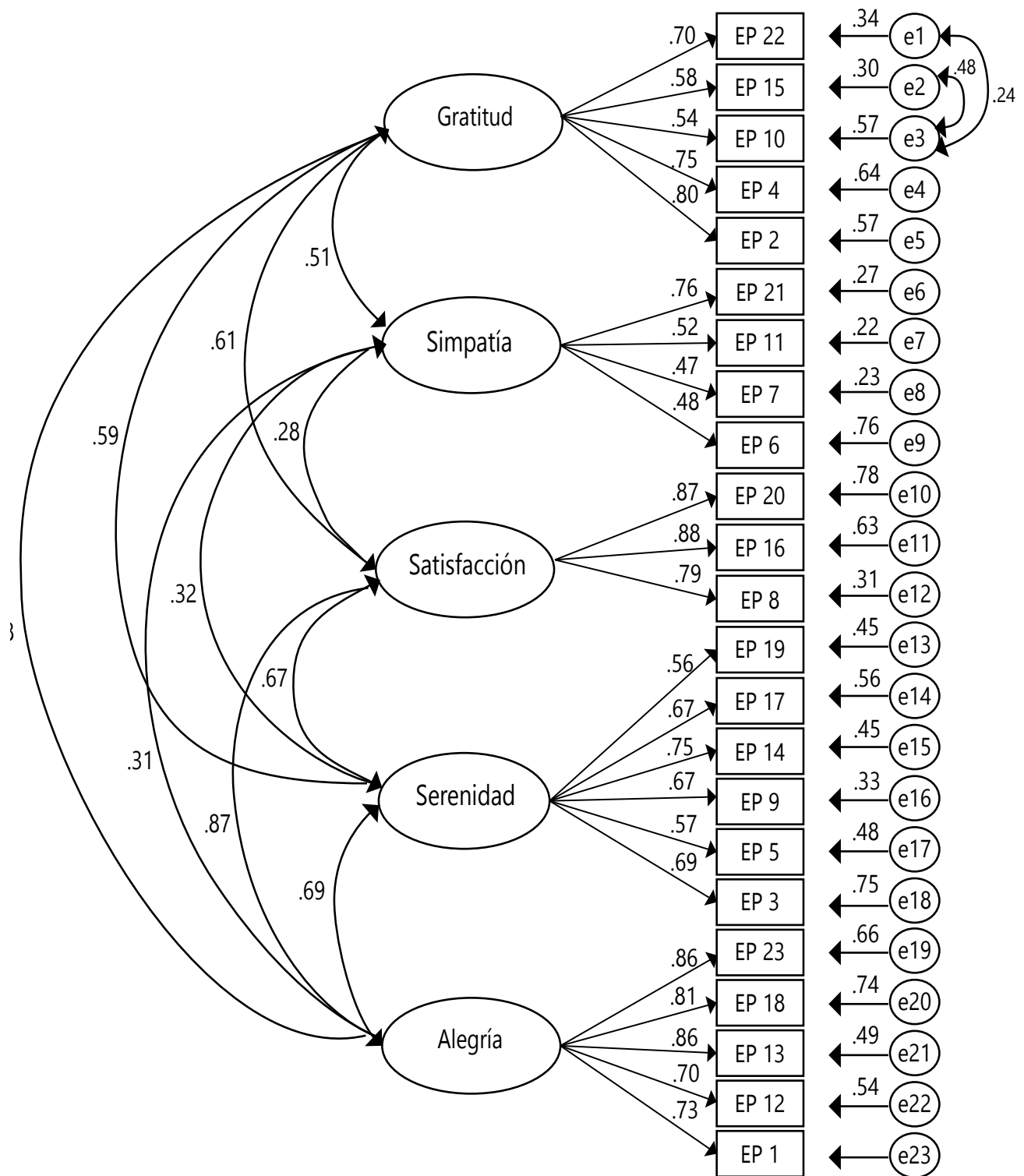
Figura 1. Modelo final para el Cuestionario de Emociones Positivas de cinco factores con coeficientes estandarizados
